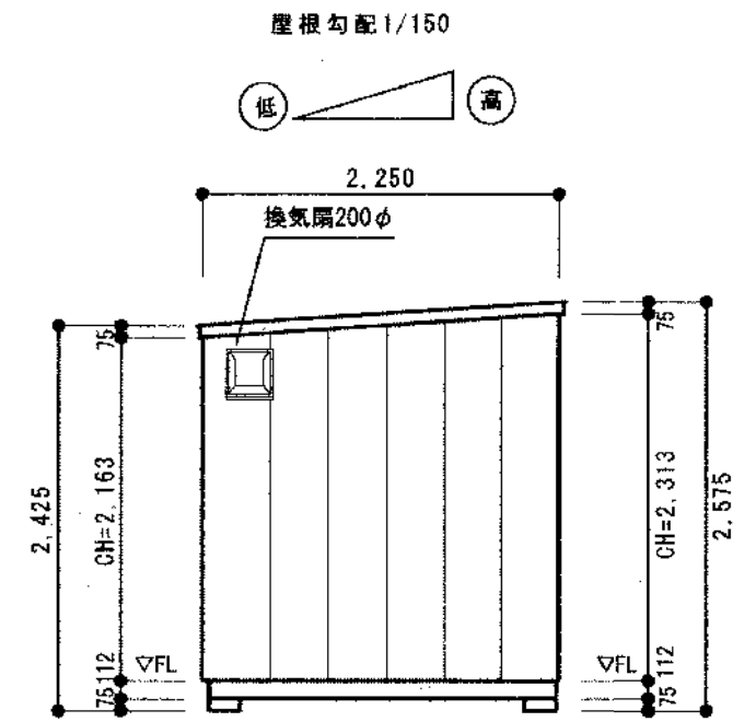
D立面図 S=1/50
