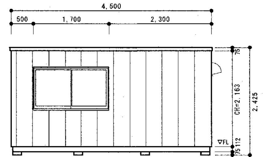
C立面図 S=1/50
