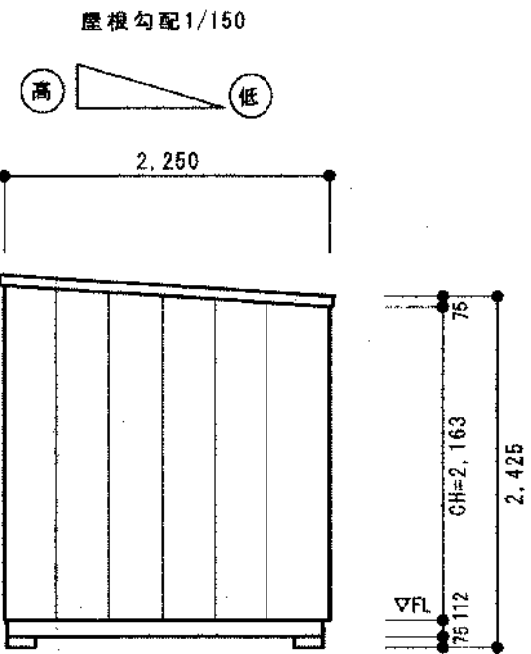
B立面図 S=1/50
