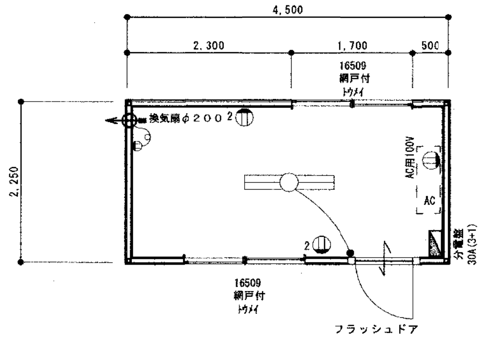
平面図 S=1/50
