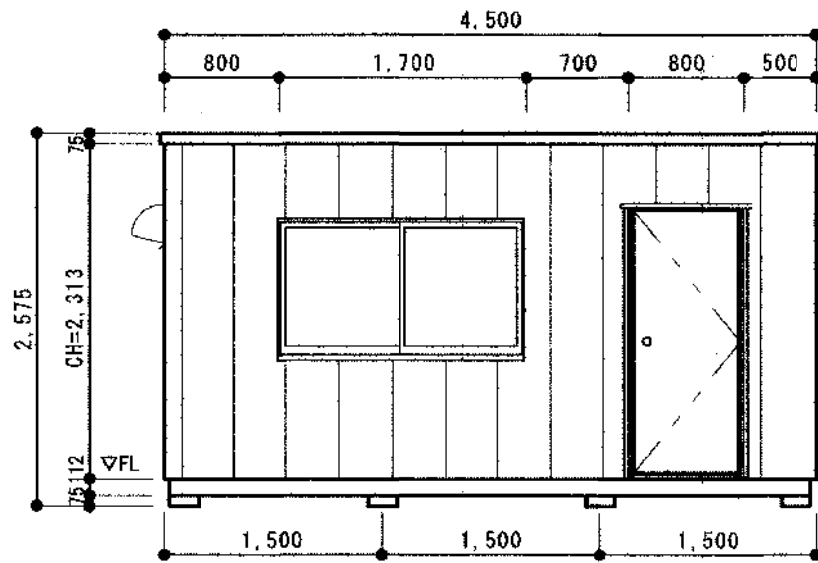
A立面図 S=1/50
